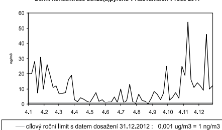
Denní koncentrace benzo(a)pyrenu v Radvanicích v roce 2011
