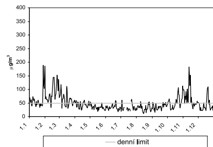
Denní koncentrace frakce prachu PM10 v Radvanicích v roce 2011
